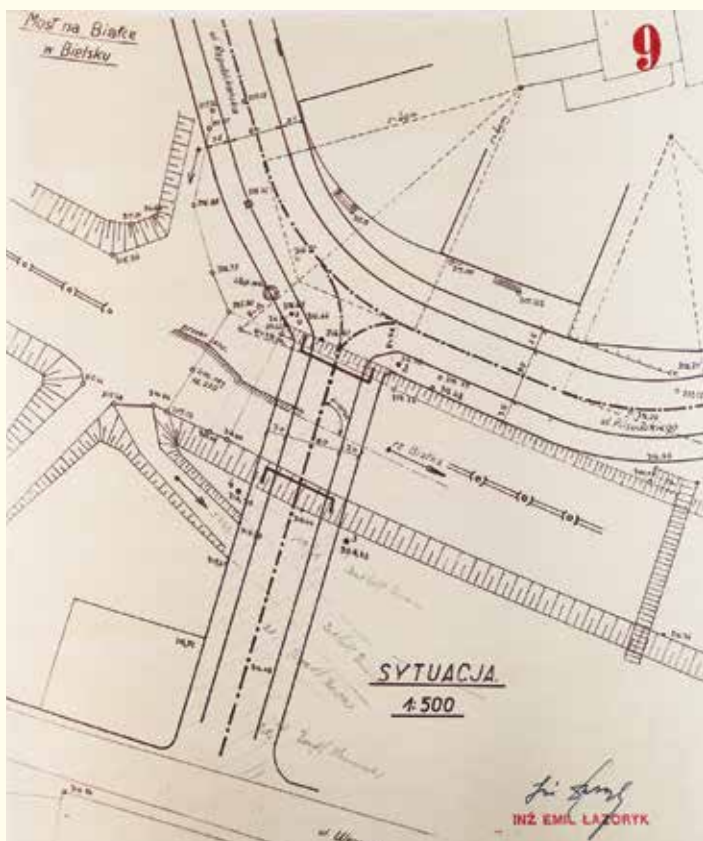
Plan sytuacyjny mostu przy ul. Republikańskiej (obecnie ul. 1 Maja)
