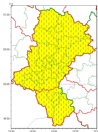
Opady marznące 2026-01-13 12:43
