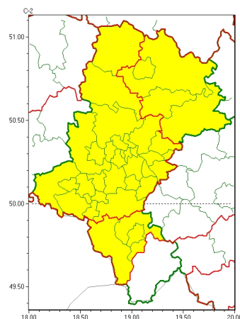
Gęsta mgła 2026-02-05 11:35
