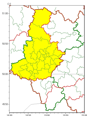
Opady marznące 2026-02-05 11:35
