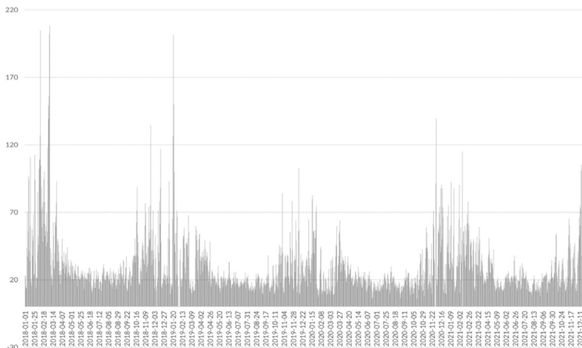
Rys. II. 63 Wartość średniego dobowego stężenia pyłu zawieszonego PM10 [ \mu\text{g}/\text{m}^3 ] na stacji pomiarowej przy ul. Zofii Kossak-Szczuckiej 19
