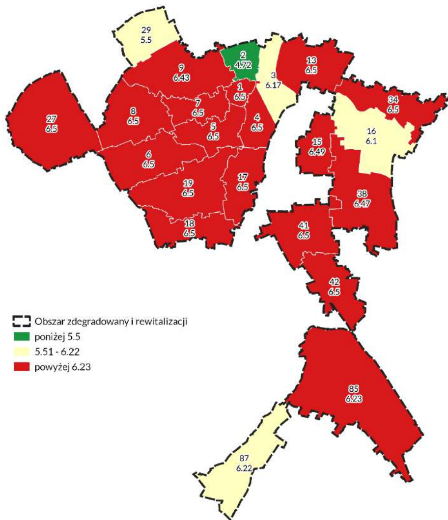
Rys. II. 66 Obszary przekroczeń średnich stężeń bezno(a)pierenu. Średnia roczna bezno(a)pierenu [µg/m³]
