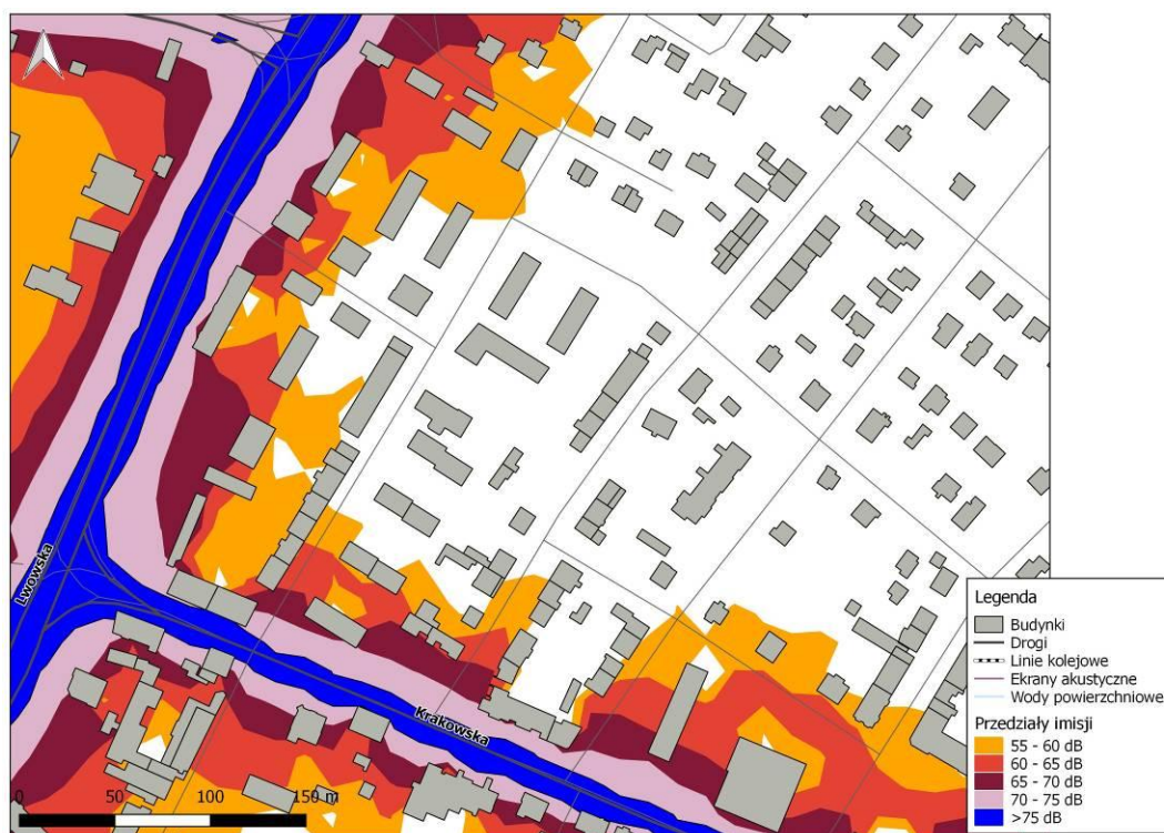
Rys. 10.13. Mapa Imisji L_{DWN} hałasu drogowego dla skrzyżowania ulic Lwowskiej i Krakowskiej od ul. Piłsudskiego do ul. Stromej przed zastosowaniem działań naprawczych
