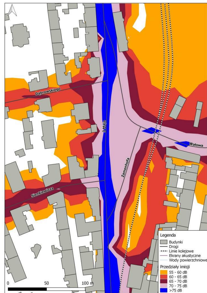
Rys. 10.30. Mapa Imisji L_{DWN} hałasu drogowego dla ul. 3 Maja na odcinku od ul. Piastowskiej do ul. Zamkowej po zastosowaniu działań naprawczych
