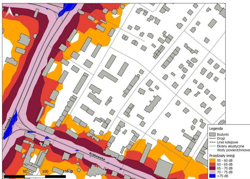
Rys. 10.14. Mapa Imisji L_{DWN} hałasu drogowego dla skrzyżowania ulic Lwowskiej i Krakowskiej od ul. Piłsudskiego do ul. Stromej po zastosowaniu działań naprawczych
