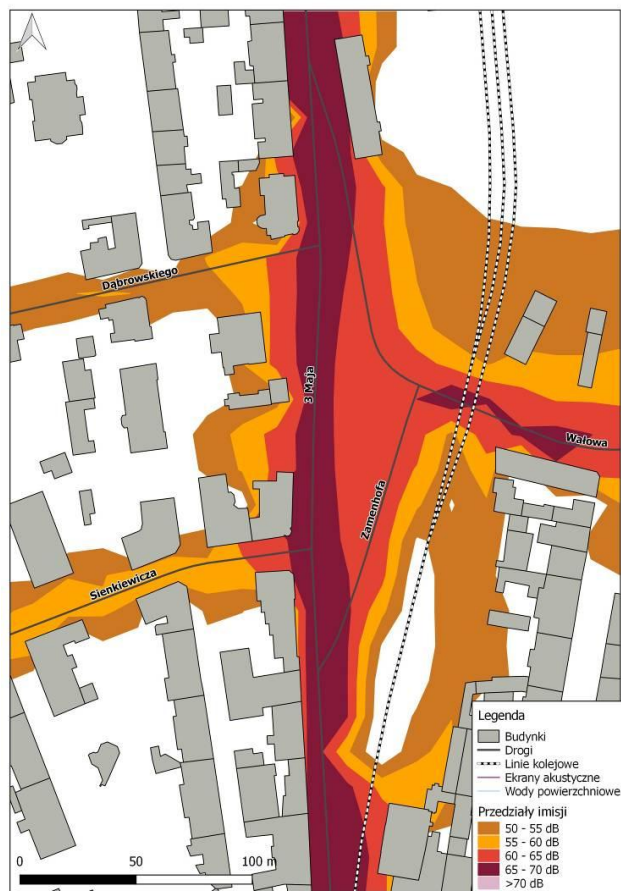
Rys. 10.32. Mapa Imisji L_N hałasu drogowego dla ul. 3 Maja na odcinku od ul. Piastowskiej do ul. Zamkowej po zastosowaniu działań naprawczych
