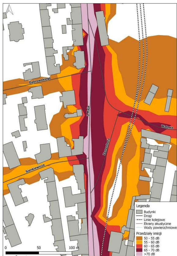
Rys. 10.31. Mapa Imisji L_N hałasu drogowego dla ul. 3 Maja na odcinku od ul. Piastowskiej do ul. Zamkowej przed zastosowaniem działań naprawczych
